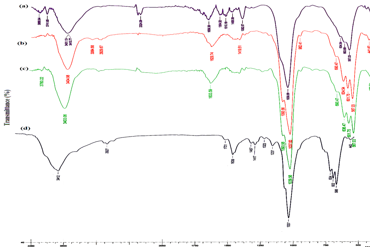
Fig. 1. FT-IR spectrum. (a) [\gamma\text{-Fe}_2\text{O}_3\text{@HAp}] , (b) [\gamma\text{-Fe}_2\text{O}_3\text{@HAp-Si(CH}_2\text{)}_3\text{Cl}] , (c) [\gamma\text{-Fe}_2\text{O}_3\text{@HAp-Si(CH}_2\text{)}_3\text{Cl@DMIM}] , (d) [\gamma\text{-Fe}_2\text{O}_3\text{@HAp-Si(CH}_2\text{)}_3\text{BF}_4\text{@DMIM}] .
