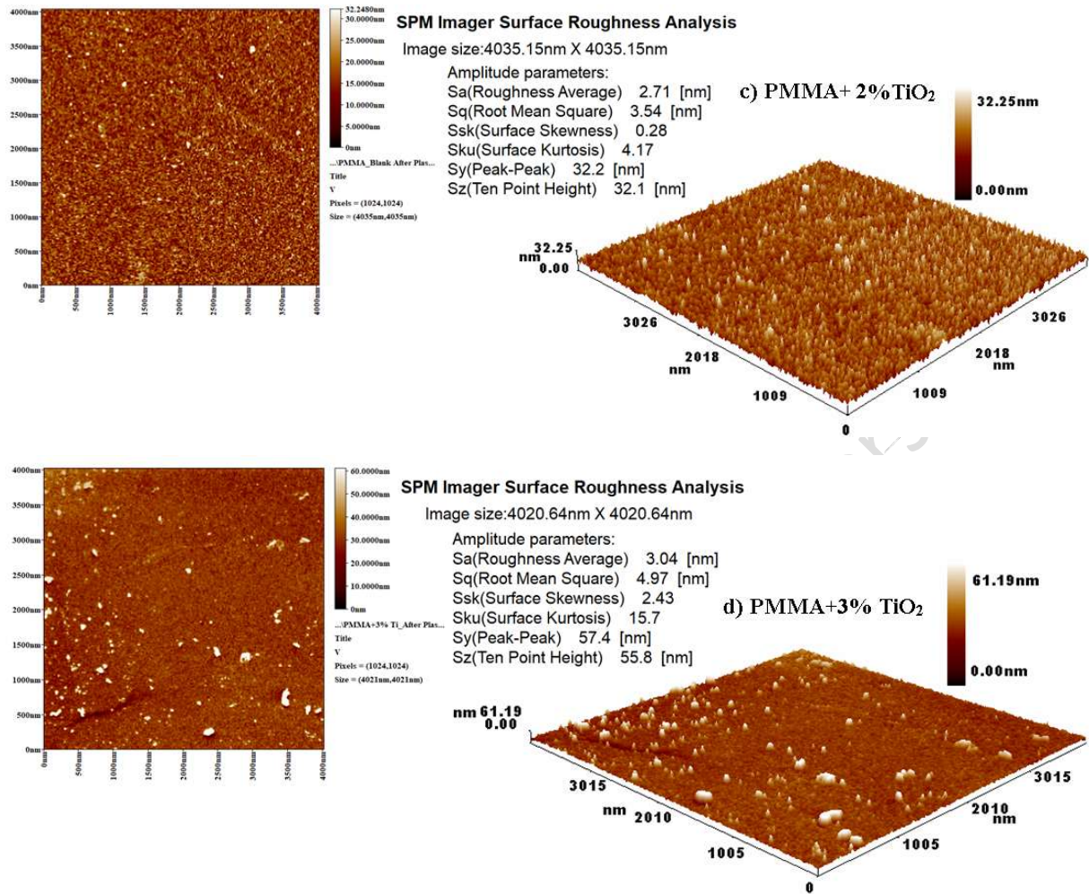
Fig. 7. AFM images for the: a) blank-PMMA, b) PMMA+1 % TiO 2 , c) PMMA+2 % TiO 2 , and d) PMMA+3 % TiO 2
